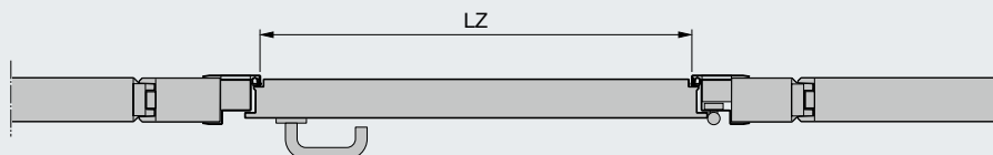
Sección horizontal
