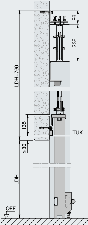
Sección vertical
